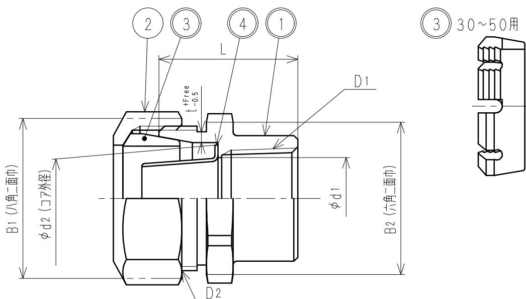
寸法表
